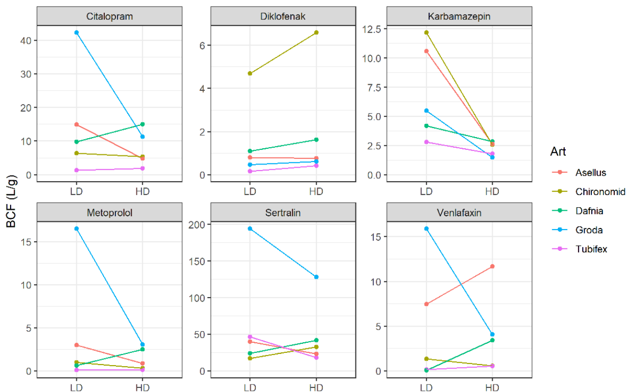
Figur 32 Beräknade biokoncentrationsfaktorer (BCF) baserat på den analyserade mängden i organismerna (ng/g våtvikt) dividerat med dosen läkemedel tillsatt till vattenfasen (ng/L), efter 28 dygns exponering för hög och låg dos.
