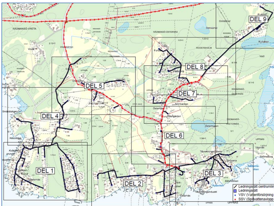
Bild 1 Förslag på ledningsdragnig i område Västernäs, Östernäs, Uppnäs m.fl.
